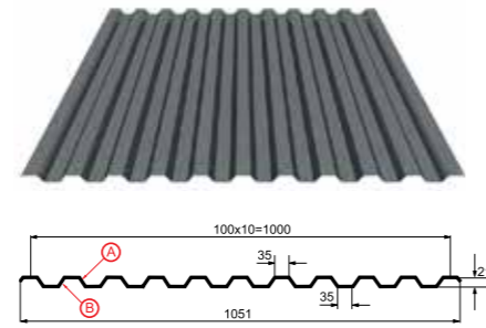
Профилированный лист С-21x1000-A Толщина материала 0.4 - 0.7 мм
