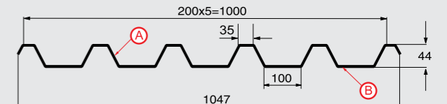
Профилированный лист С-44x1000-А Толщина материала 0.45 - 0.8 мм
