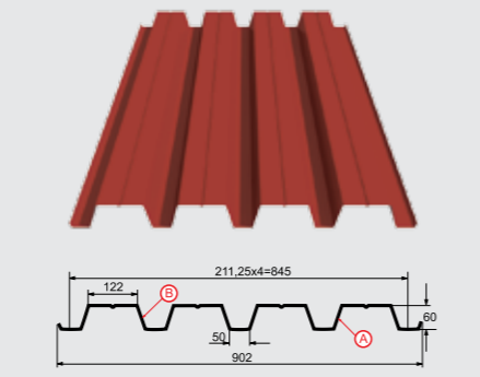
Профилированный лист Н-60x845-A,B Толщина материала 0.5 - 1.0 мм
