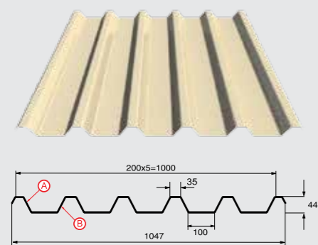
Профилированный лист С-44x1000-A Толщина материала 0.45 - 0.8 мм
