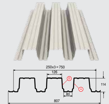
Профилированный лист Н-114x750-A,B Толщина материала 0.7 - 1.0 мм
