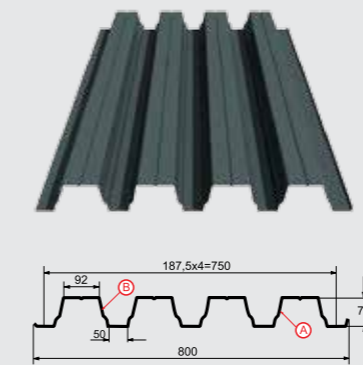
Профилированный лист Н-75x750-A,B Толщина материала 0.65 - 1.0 мм
