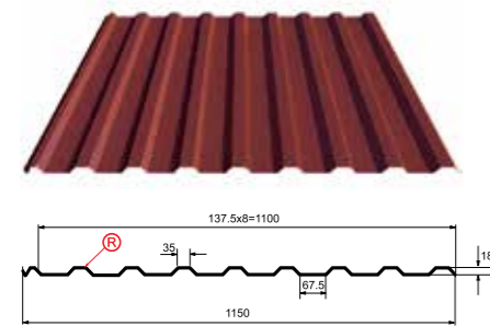
Профилированный лист МП-20x1100-B, R Толщина материала 0.4 - 0.8 мм
