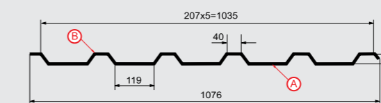
Профилированный лист МП-35x1035-А Толщина материала 0.45 - 0.9 мм
