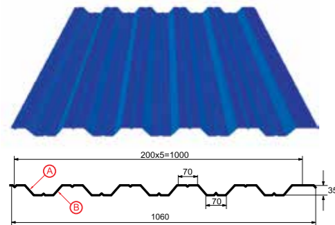
Профилированный лист НС-35x1000-A Толщина материала 0.45 - 0.9 мм
