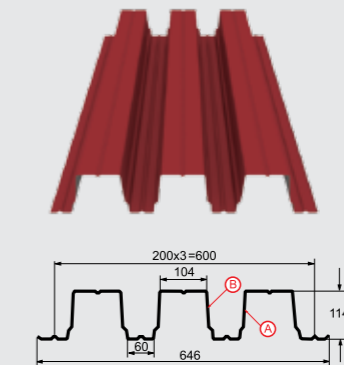
Профилированный лист Н-114x600-A,B Толщина материала 0.7 - 1.0 мм
