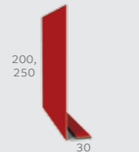
Планка карнизного свеса 200x30x2000, 250x30x2000
