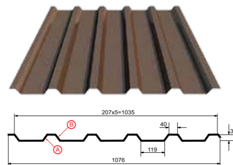
Профилированный лист МП-35x1035-B Толщина материала 0.45 - 0.9 мм
